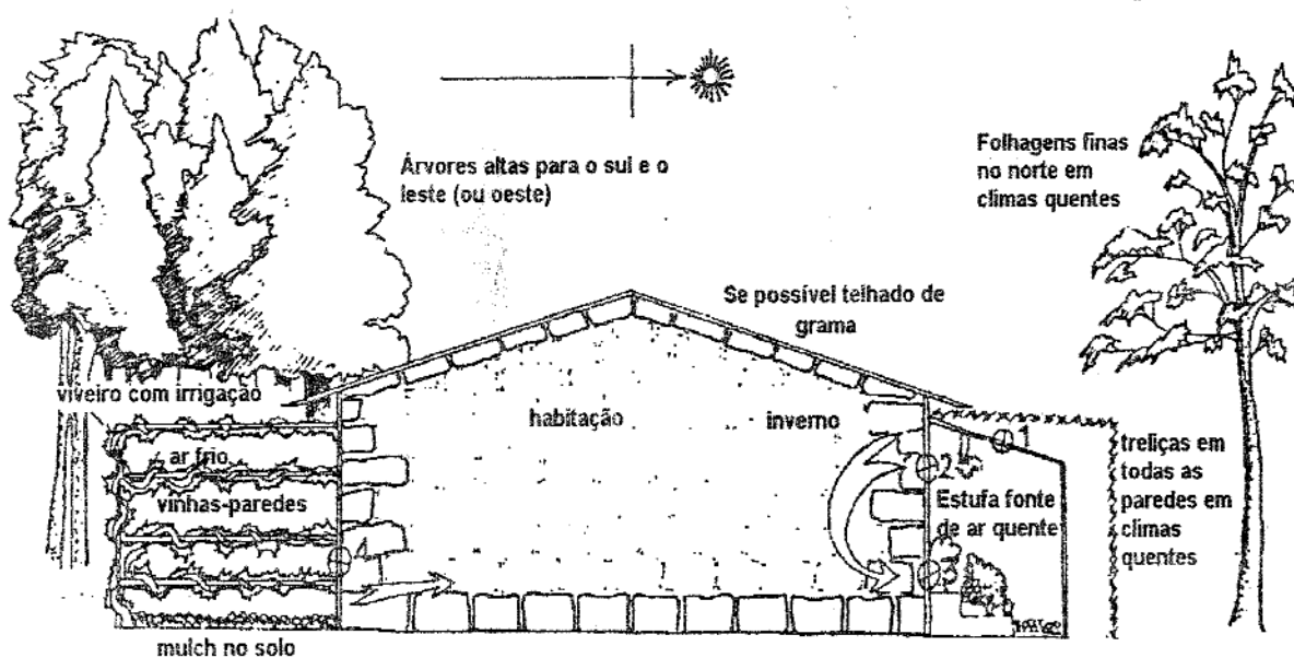
Figura 4.9 Ar frio circula do viveiro para a casa, sugado pela estufa. Vinhas caducifólias (uvas) estão no lado do sol, enquanto que vinhas perenifólias estão no lado da sombra.
