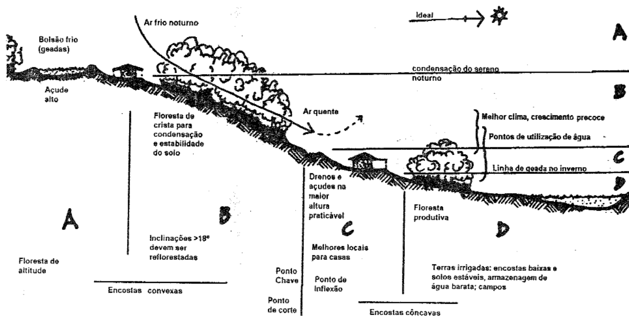
Figura 1.6 Análise da encosta e o plano para o sítio em relação ao aspecto influenciam muito no posicionamento do acesso, suprimento de água, florestas e plantios em geral (zonas úmidas).
