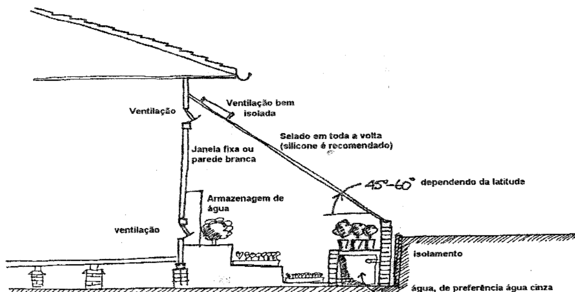
Figura 4.8 Uma estufa no lado do sol ajuda com o aquecimento da casa, particularmente em climas frios. Ventilação é essencial para o controle climático da casa, tanto no inverno quanto no verão.
