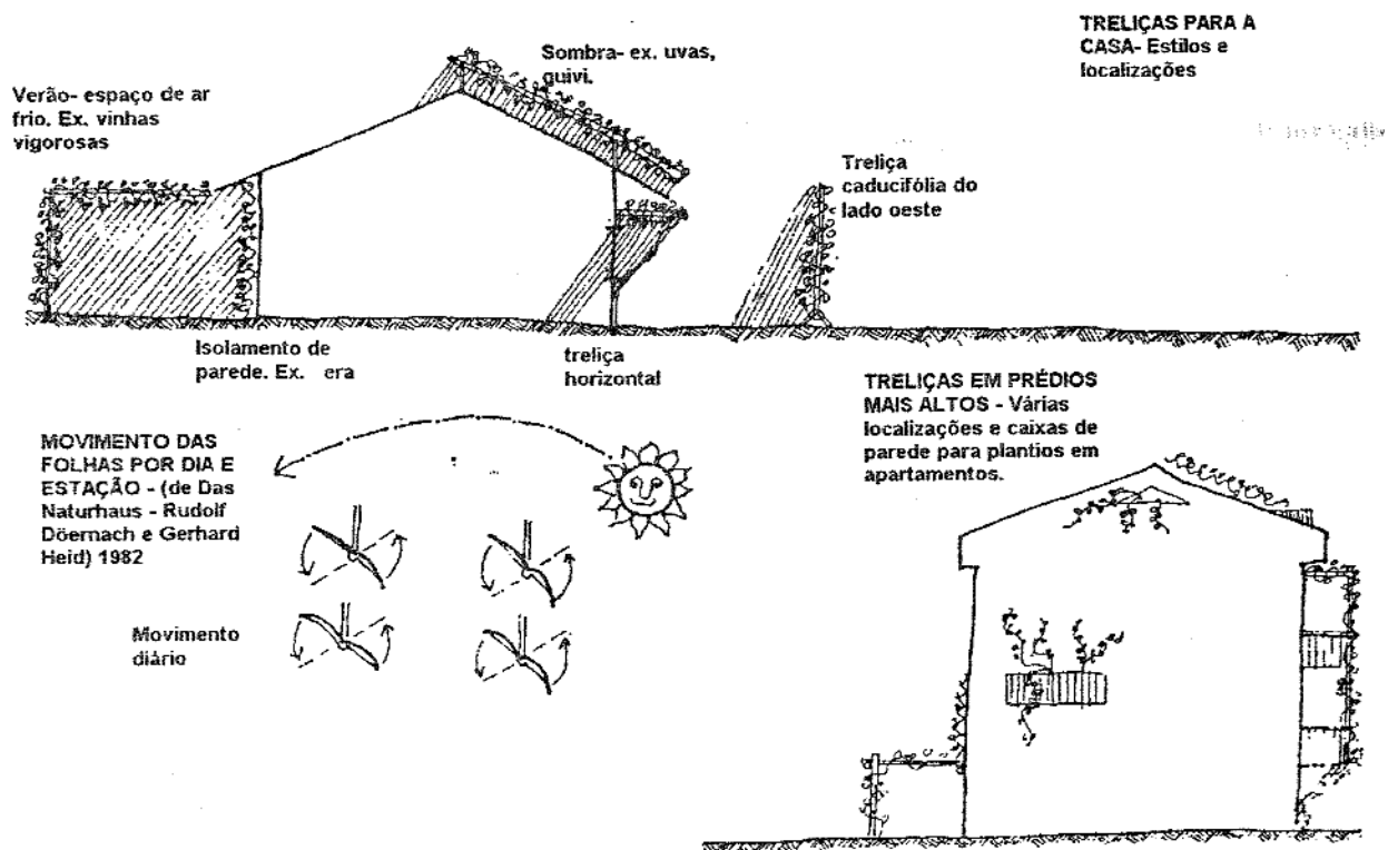
Figura 4.7 Trelças com vinhas em edificações permitem sombra no verão. Se as vinhas são caducifólias, permitem a luz solar penetrar a casa durante o inverno. A cozinha e o banheiro partilham os canos de água e deveriam ser posicionados juntos.
