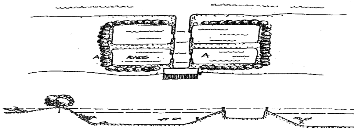
Figura 7.22 Plano e corte para tanques de maré.
