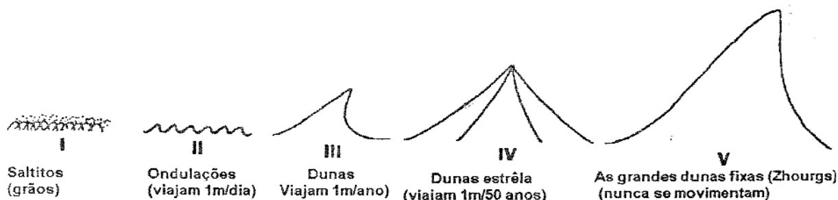
Figura 3.5 Dunas de areia formam cinco ordens de tamanho, comuns a uma grande variedade de fenômenos.
