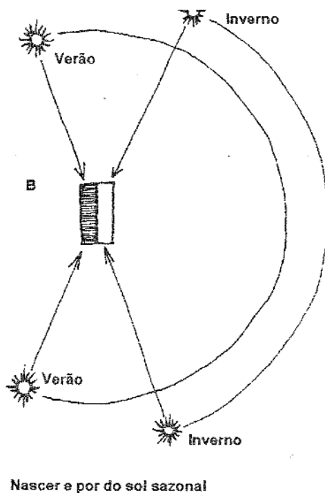
Figura 2.1 A direção do sol, e sua altura em relação ao horizonte durante o ano, afetam o projeto da casa e das comunidades de plantas.
