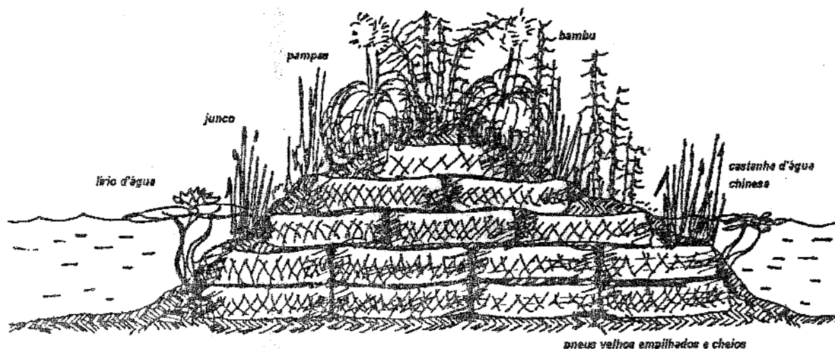
Figura 7.19 Ilha de pneus para tanque de água fresca
