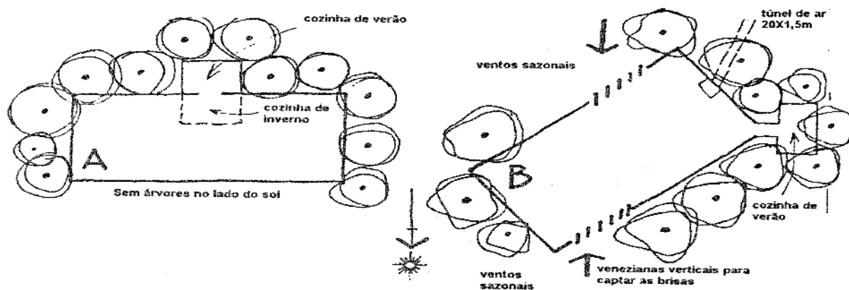
Figura 4.11 Posicionamento de casas em (A) subtropical, onde a orientação existe em relação ao sol, (B) nos trópicos, onde a orientação é em direção às brisas refrescantes e para sombrear todo o perímetro.
