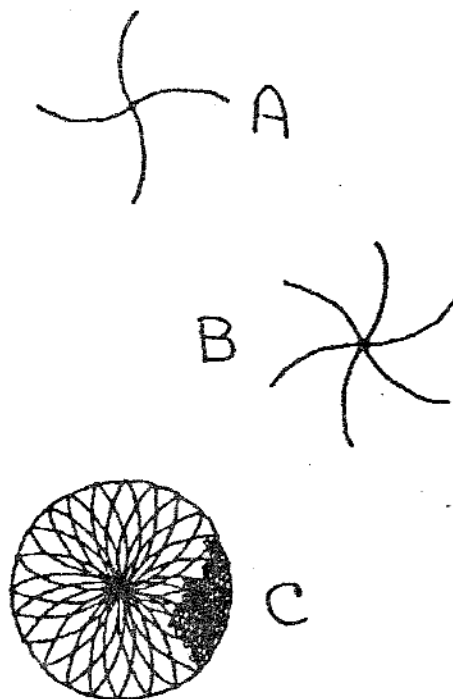
Figura 3.3 - Modelos de fluxo de seiva
