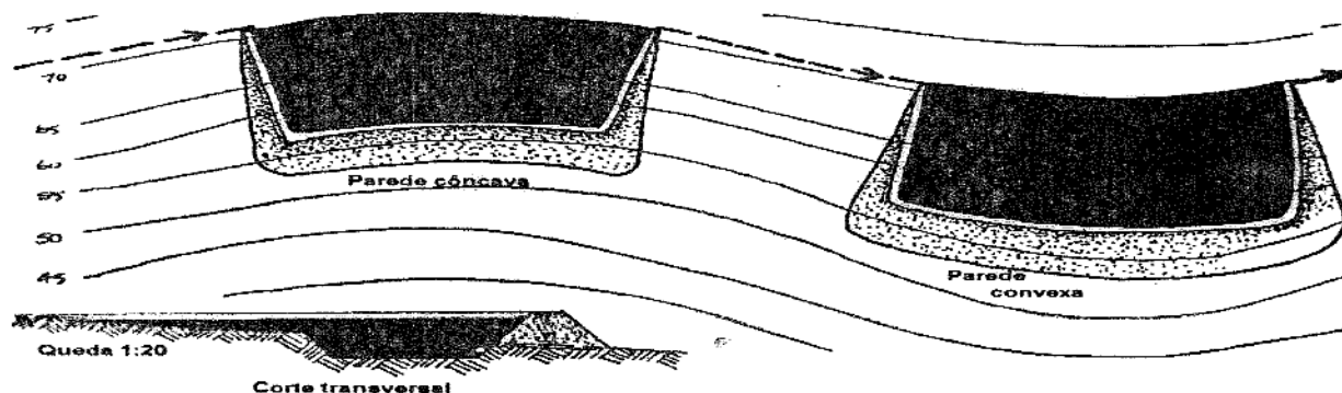
Figura 2.28 Açudes em curva de nível são viáveis em encostas de 8 graus ou menos, como parte da série de açudes da fazenda.
