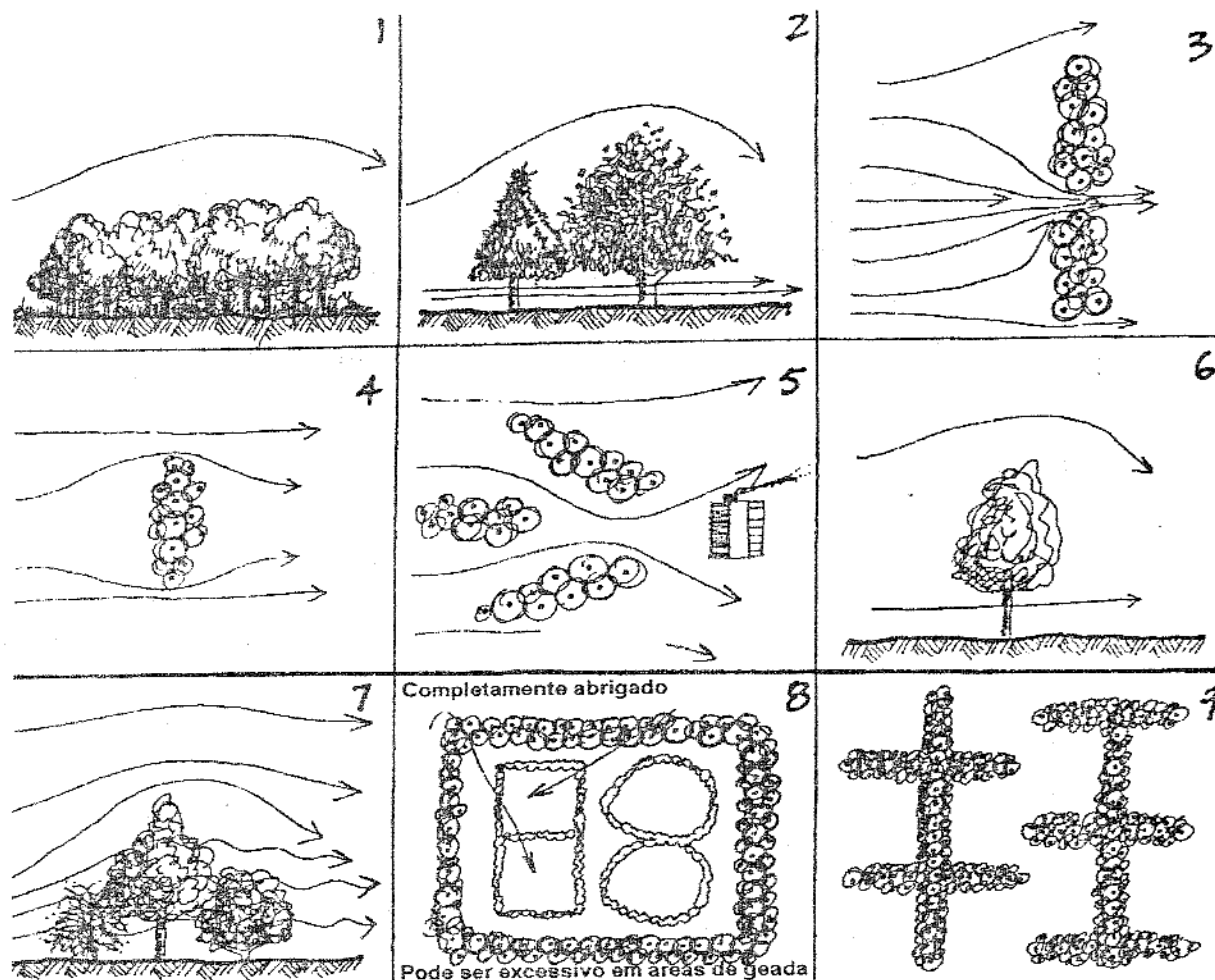
Figura 2.15 QUEBRA VENTOS QUE NÃO FUNCIONAM: (1) muito largo, (2) sem galhos baixos, acelera o vento, (3) lacunas aceleram o vento (efeito Venturi), (4) muito estreito, (5) não perpendicular ao vento, (6) somente uma carreira de árvores.
